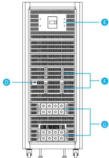
(后视图)
