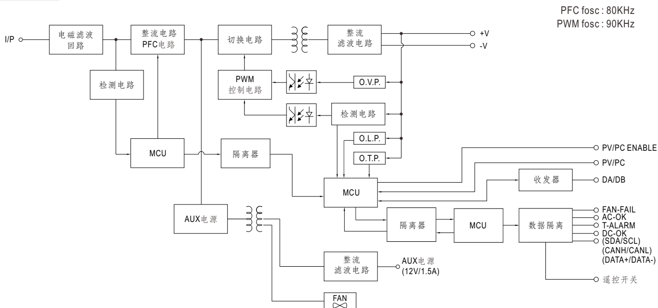
■ 方框图
