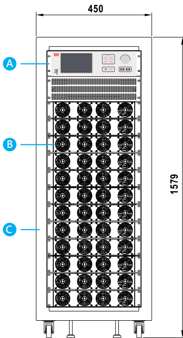
(正视图)
